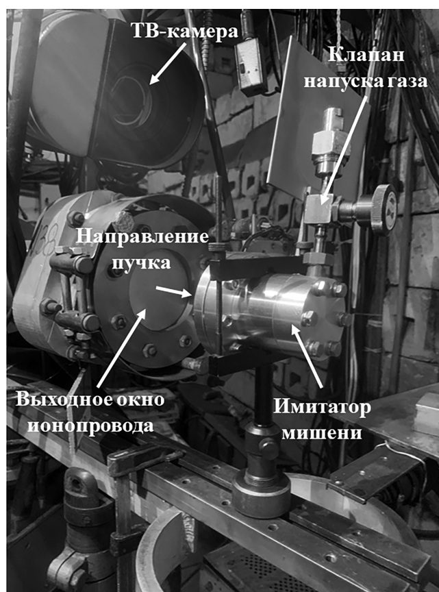
Рис. 2. Место расположения имитатора мишени.
