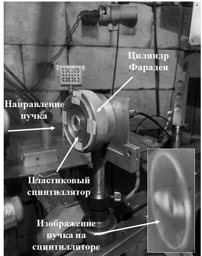
Рис. 4. Место расположения цилиндра Фарадея и изображение пучка на пластиковом сцинтилляторе, зарегистрированное камерой.
