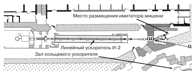
Рис. 1. Схема выводных каналов ускорителя И-2 и место расположения имитатора мишени.
