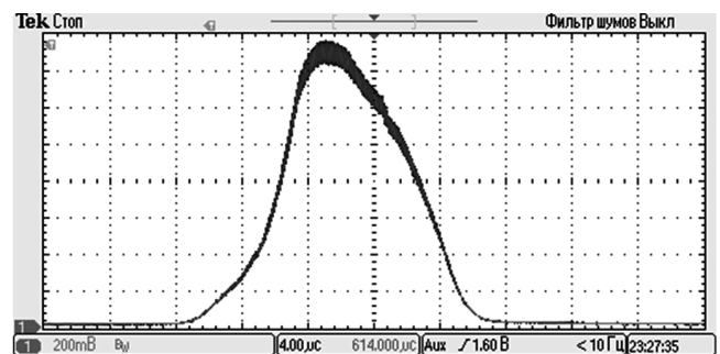
Рис. 5. Осциллограмма выходного сигнала с цилиндра Фарадея.
