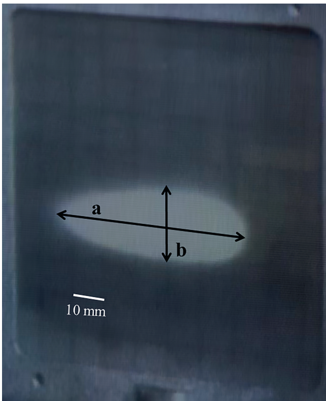
Рис. 3. Изображение пучка на сцинтилляторе из керамики.
