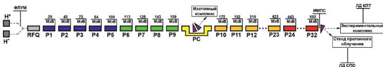
Рис. 1. Схема линейного ускорителя ИЯИ РАН: ФЛУМ – флуоресцентный монитор; ИМПС – ионизационный монитор поперечного сечения; ЛД СПО – люминесцентная диагностика стенда протонного облучения; ЛД КПТ – люминесцентная диагностика; RFQ – резонатор с пространственно-однородной квадрупольной фокусировкой; P – резонатор.
