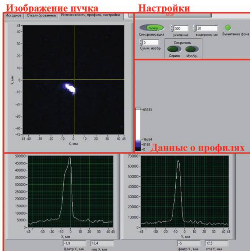
Рис. 3. Вкладка интерфейса программы обработки изображения с люминесцентного экрана КПТ.
