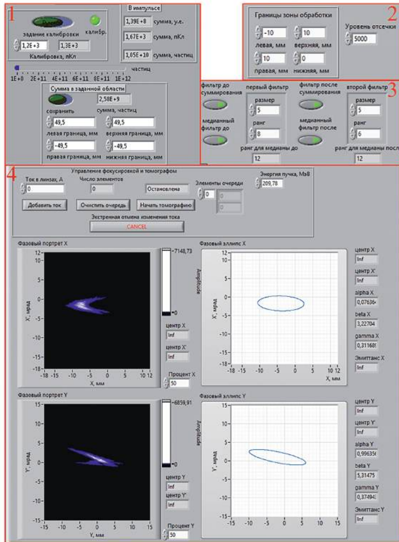
Рис. 4. Интерфейсы дополнительных модулей: 1 – модуль расчета заряда, 2 – модуль выбора области интереса, 3 – модуль ранговой фильтрации, 4 – модуль онлайн-томографии.
