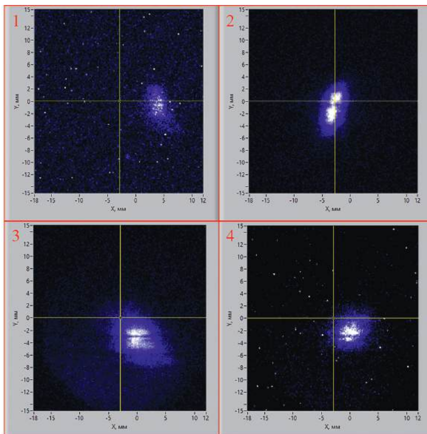
Рис. 5. Изображения пучков с разными параметрами с ИМПС: 1 – пучок H^+ с импульсным током 12 мкА, длительностью 20 мкс, энергией 158 МэВ; 2 – пучок H^- с импульсным током 1.5 мА, длительностью 47 мкс, энергией 100 МэВ; 3 – пучок H^+ с импульсным током 7 мА, длительностью 100 мкс, энергией 267 МэВ; 4 – пучок H^+ с импульсным током 10 мА, длительностью 0.25 мкс, энергией 267 МэВ.
