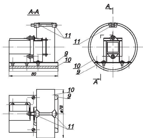
Рис. 5. Конструкция линзы.
