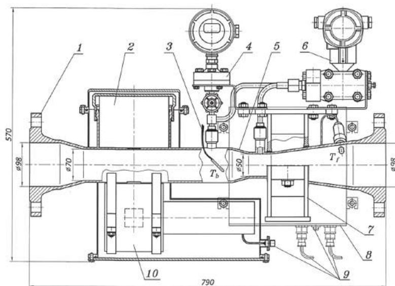
Рис. 1. Конструкция бессепарационного трехфазного расходомера “нефть–вода–газ” горизонтальной ориентации DN 100: 1 – соединительный фланец, 2 – двухизотопный гамма-источник, 3 – платиновые датчики Pt1000 температуры потока T_f и корпуса T_b , 4 – датчик давления, 5 – сужающее устройство 70/50 мм, 6 – датчик перепада давления, 7 – крепежная рама, 8 – взрывобезопасный корпус электроники, 9 – разъемы датчиков, гамма-детектора, питание 24 В и Ethernet, 10 – спектрометрический гамма-детектор.
