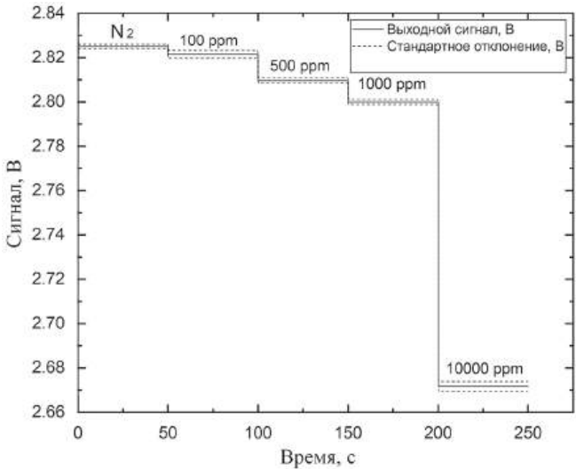
Рис. 7. Результаты тестирования течеискателя при разных концентрациях метана.
