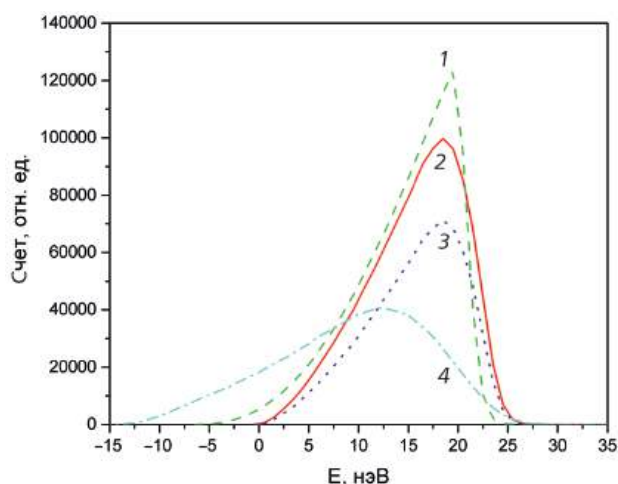
Рис. 3. Спектр УХН в различные моменты времени: 1 – 650 с, 2 – 700 с, 3 – 1000 с, 4 – при регистрации на детекторе. Отсчет энергии ведется от дна ловушки в горизонтальном положении ( \theta_{\text{trap}} = 0^\circ ).
