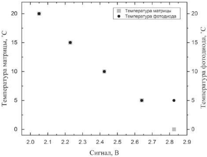
Рис. 6. Зависимость уровня выходного сигнала от температур, установленных на матрице и фотодиоде.
