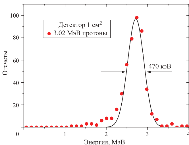
Рис. 5. Энергетическое разрешение детектора при регистрации протонов с энергией 3 МэВ (замедленных в алюминиевой фольге толщиной 10 мкм). Приведены данные для диода с площадью чувствительной поверхности 1 \text{ см}^2 .
