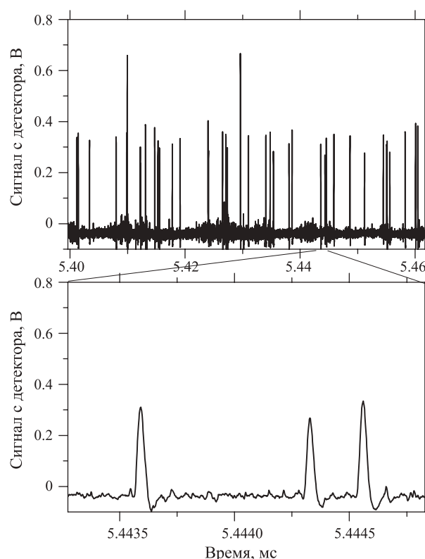
Рис. 4. Пример фрагмента осциллограммы, полученной с детектора на основе диода площадью 1 \text{ см}^2 .
