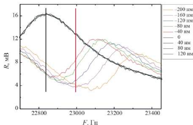
Рис. 1. Резонансные кривые кварцевого осциллятора R(F) при различных значениях его смещения ( h ) над поверхностью подложки. Частота резонанса свободно колеблющегося кварцевого резонатора с прикрепленным капилляром F = 22\,840 Гц отмечена вертикальной черной линией. Оптимальная частота для корректной работы системы обратной связи АСМ F = 23\,000 Гц отмечена вертикальной красной линией.
