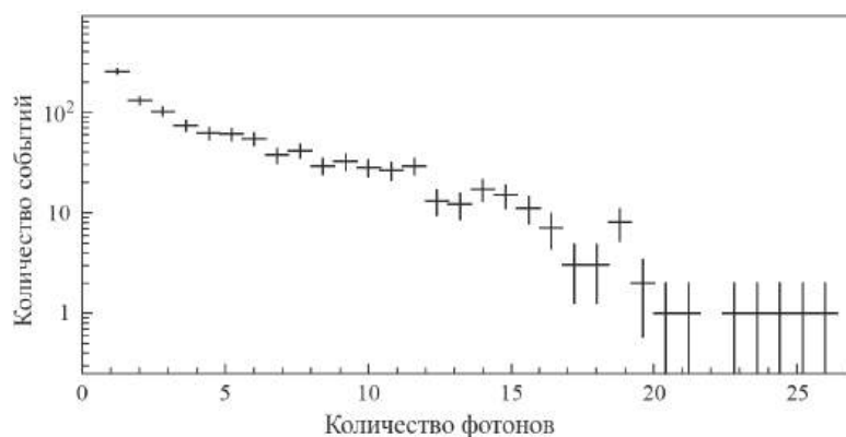
Рис. 5. Зависимость количества событий от величины светового сигнала.
