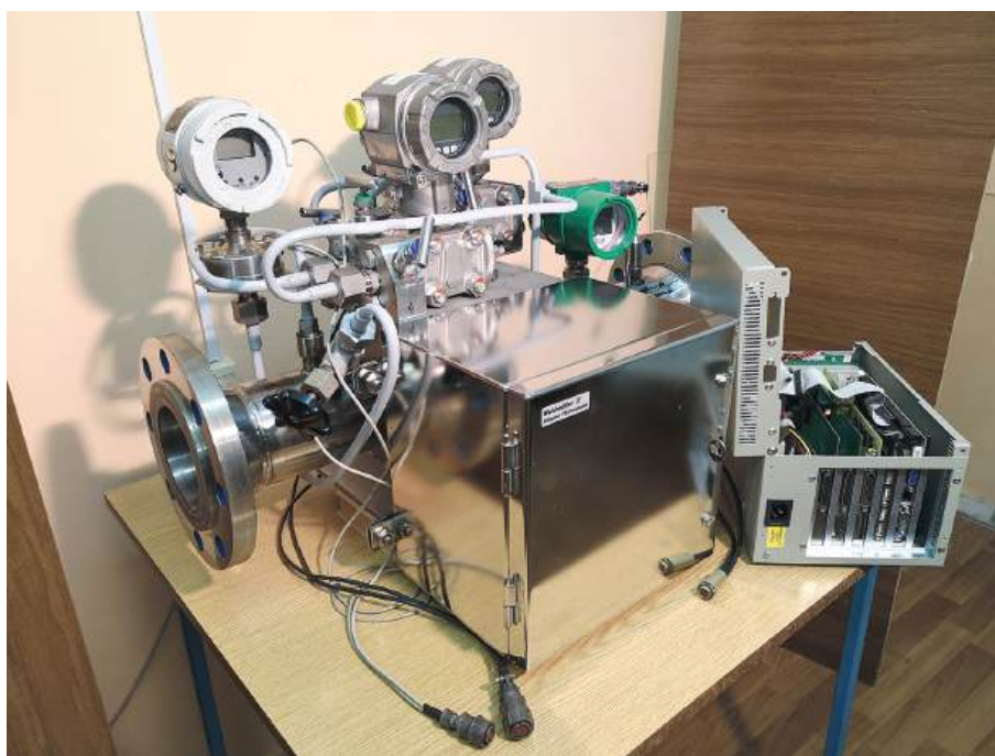
Рис. 8. Универсальный двухфазный расходомер DN 100: комбинация пары конических сужающих устройств 98/70 и 70/50 мм, камертонного плотномера 804 (справа от датчиков перепада давления), тонкопленочных датчиков температуры Pt1000 [17] и измерительной системы на базе промышленного компьютера (ПК).
