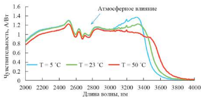
Рис. 4. Зависимость чувствительности фотодиода от длины волны.
