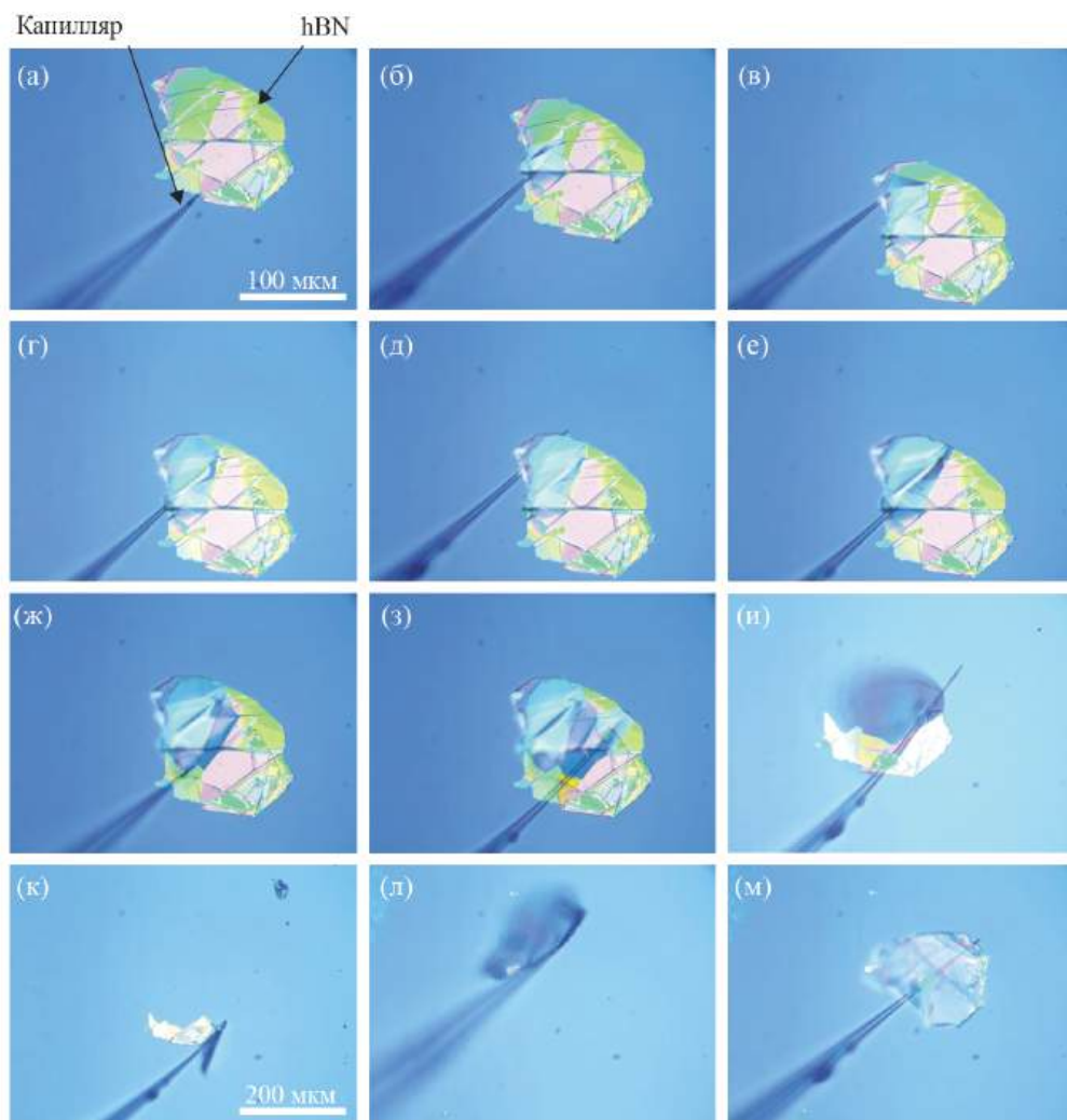
Рис. 5. Этапы процесса перемещения пластины hBN большого (более 100 микрон) размера: а–д – подведение зонда под лист, е–л – отделение листа от поверхности, м – лист hBN лежит на капилляре, т.е. подготовлен для перемещения на другое место данной подложки или к переносу на другую подложку. Масштабы на рис. а–и и на рис. к–м совпадают.
