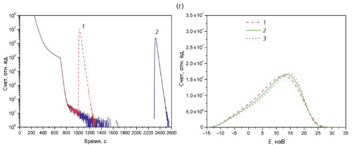
Рис. 5. Результаты моделирования измерений с разными углами мониторингирования: а – 2.5^\circ , б – 5^\circ , в – 7.5^\circ , г – 10^\circ . Слева – временная диаграмма для разных времен удержания, когда время поворота ловушки на 180^\circ составляет 90 с: 1 – короткое время удержания, 2 – длинное. Справа – соответствующий спектр нейтронов при регистрации на детекторе после короткого времени удержания со следующими временами поворота ловушки на 180^\circ : 1 – 90 с, 2 – 135 с, 3 – 180 с.
