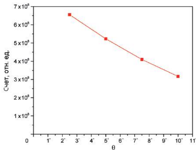
Рис. 6. Зависимость количества нейтронов в сливе после короткого времени удержания от угла мониторингирования. Время поворота ловушки на 180^\circ составляет 90 с.
