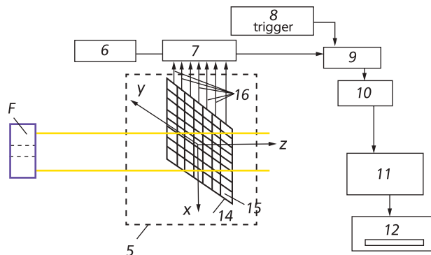
Рис. 5. Схема проведения эксперимента [1] на “правой” части установки: F – регулируемая диафрагма из материала ПОВ-40, которая “вырезает” нужную часть пучка нейтронов.
