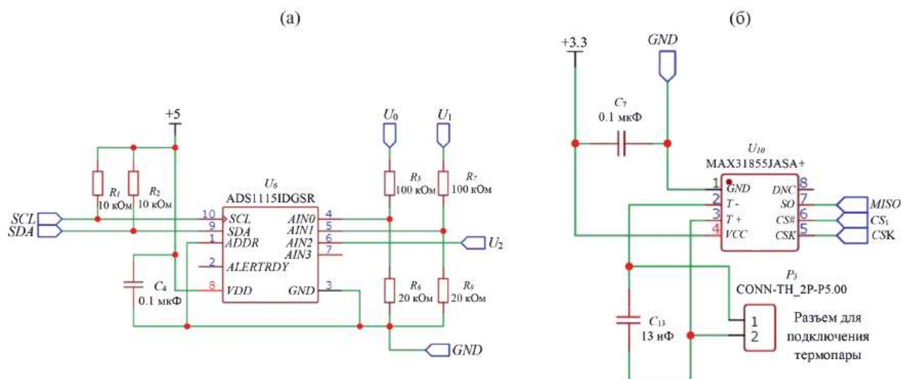
Рис. 6. Аналого-цифровой преобразователь (а) и преобразователь сигнала термодатчика (б).
