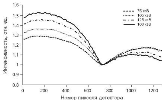
Рис. 9. Распределение эффективной энергии рентгеновского излучения по детектору относительно пятна со сниженной интенсивностью для источника 615 кВ и симметричной электродной системой. Распределение соответствует линии пикселей, отмеченной стрелкой на рис. 8.
