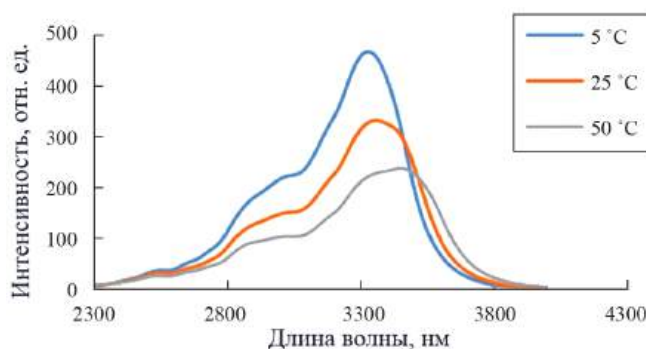
Рис. 3. Зависимость интенсивности излучения матрицы от температуры.
