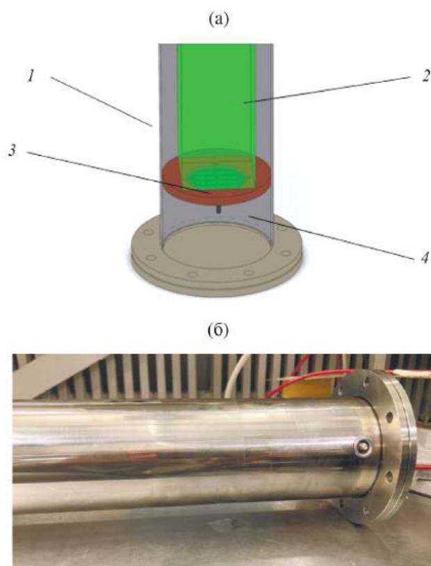
Рис. 2. а) 3D-модель сборки со стороны матрицы SiPM: 1 – герметичный кожух, 2 – сцинтиллятор, 3 – матрица SiPM из 16 штук, 4 – фиксирующая вставка. б) Фотография экспериментального образца (со стороны матрицы SiPM).
