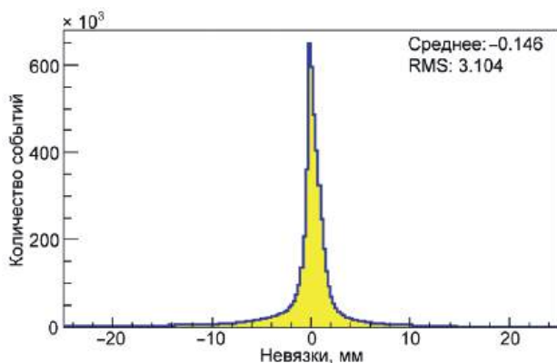
Рис. 13. Распределение невязок.
