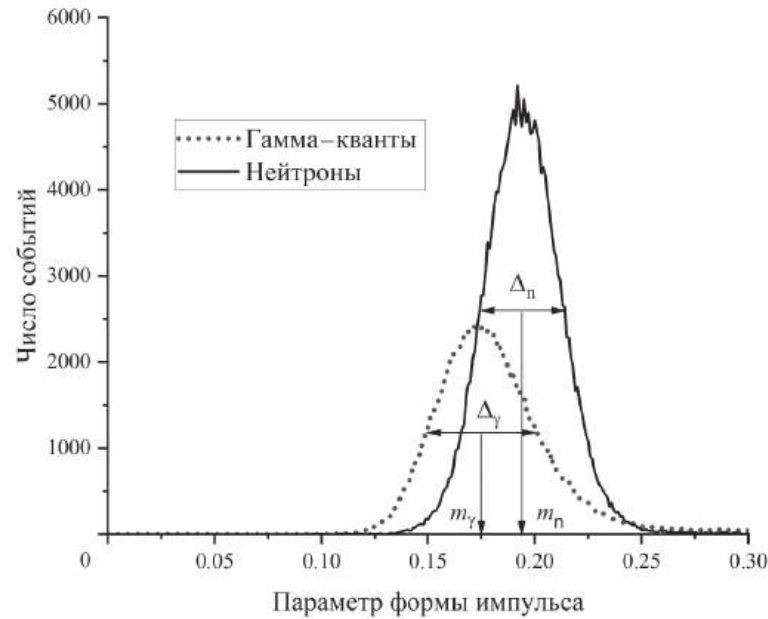
Рис. 5. Распределения импульсов по значению параметра PSP для нейтронов и γ-квантов.
