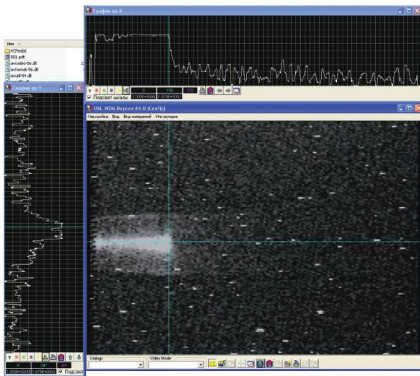
Рис. 1. Рабочий кадр процесса точного наведения траектории пучка протонов с энергией 100 МэВ в водном фантоме детектора ЦДПИ во время сеанса в 2023 году, при котором проходили измерения K_{\text{осл}} . Окно программы OSC-16 с энергией пучка 100 МэВ.
