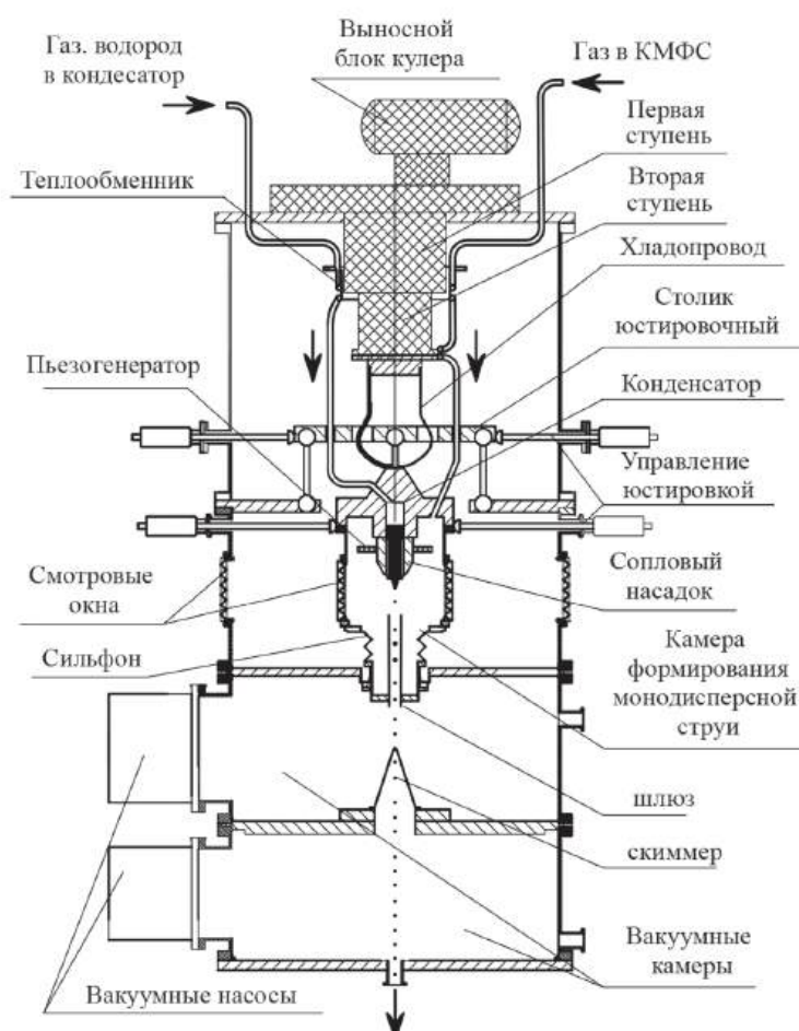
Рис. 2. Схема криостата прототипа криогенной корпускулярной водородной мишени.
